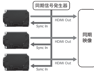
複数カメラ利用時の仕組み（例）
